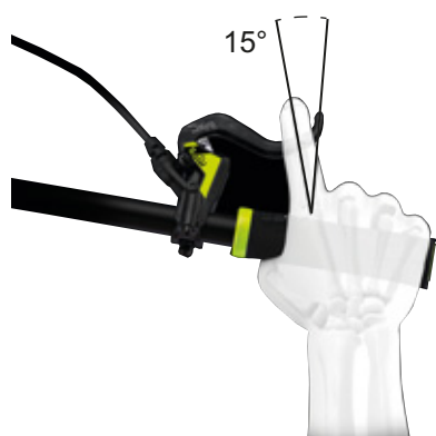
Figur 118: Bremsegrebets position
