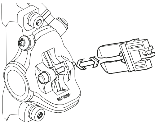
Figur 62: Fastgørelse af transportsikring
