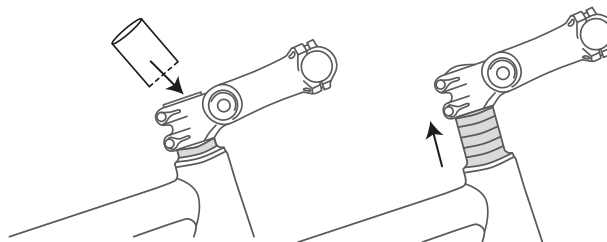
Figur 112: Forhøjning af Ahead-frempind ved at montere afstandsringe (spacers)
