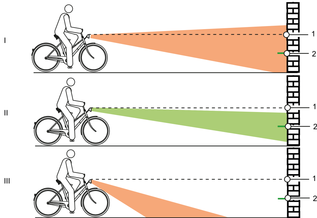
Figur 187: For højt (1), korrekt (2) og for lavt (3) indstillet lys
