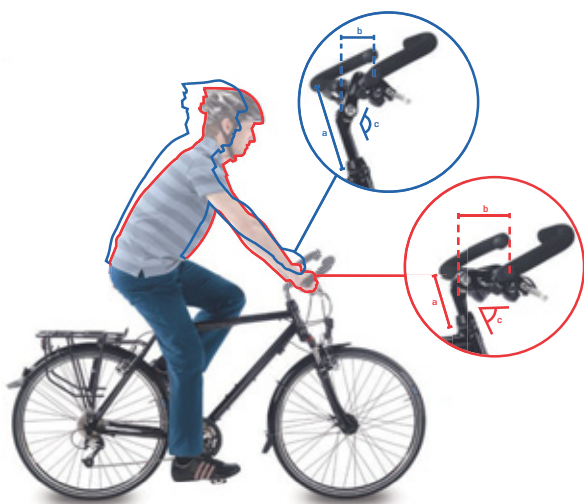
Figur 114: Position for citybike (blå) og trekkingcykel (rød) med vinkelændring
