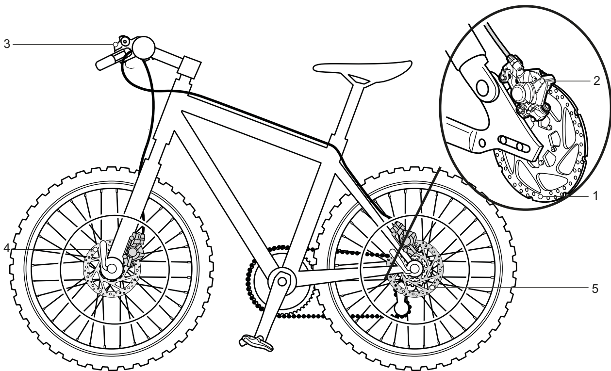
Figur 27: Bremsesystem med skivebremse, eksempel
