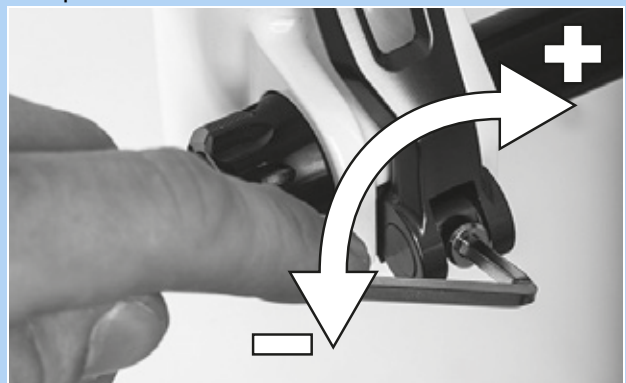
Figur 194: Indstilling af hurtigbespændingens spændekraft
