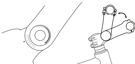
Figur 113: Forskellige versioner af vinkeljusterbare frempinde
