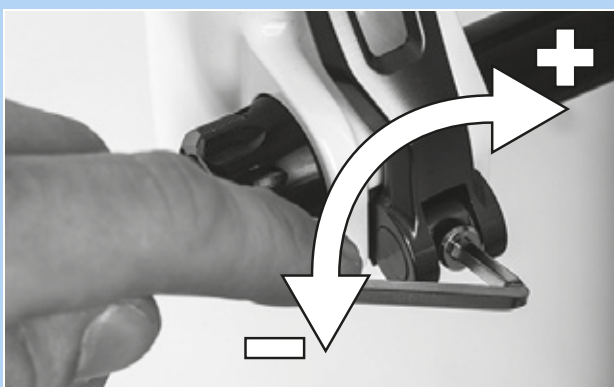
Figur 74: Indstilling af hurtigbespændingens spændekraft
