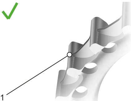
Figur 177: Optimal tandprofil
