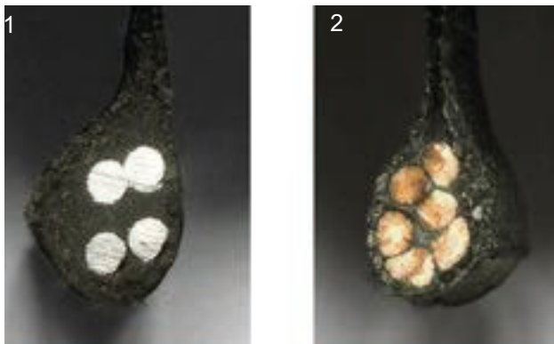
Figur 19: Stålkerner (1) og kevlarkerner (2)
