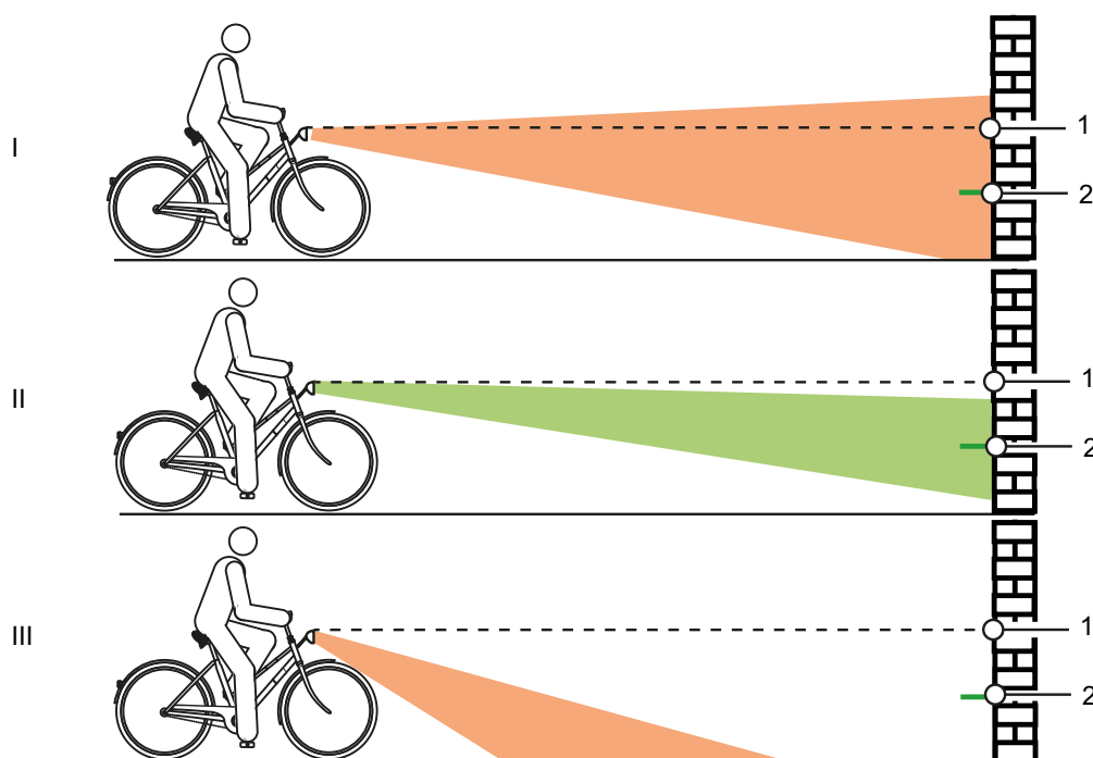
Figur 129: For højt (1), korrekt (2) og for lavt (3) indstillet lys
