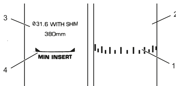
Figur 103: Detaljeret visning af sadelpind, eksempler på markering af minimumsdybden
