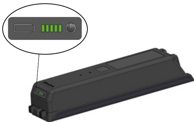
Figur 59: Placering af ladetilstandsindikator (batteri)
