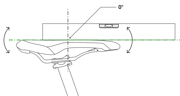
Figur 106: Vandret sadelhældning med 0° hældning i sadelmidten
