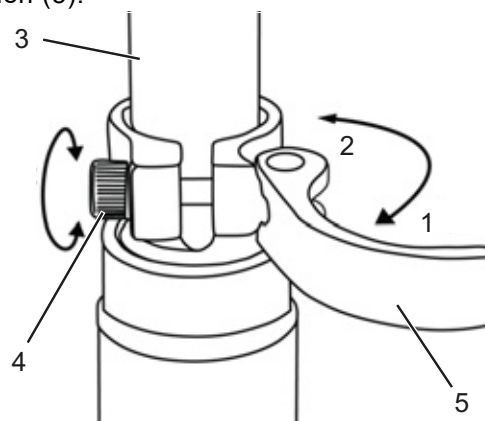
Figur 102: Løsning af sadelpindens hurtigbespænding
