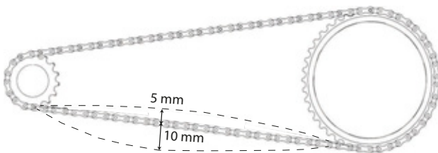
Figur 166: Eksempel på kontrol af kædestramning: 5 mm opad, 10 mm nedad = 15 mm afvigelse
