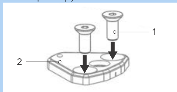
Figur 81: Indsætning af skruerne med undersænket hoved i basispladen
