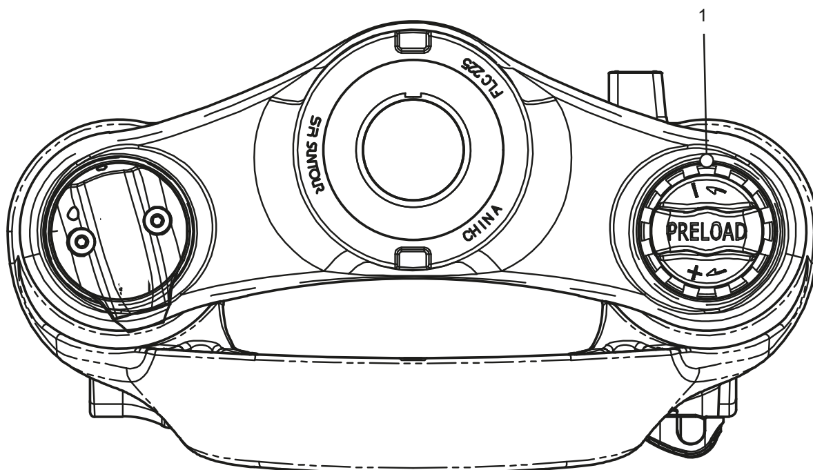
Figur 123: Indstillingshjul for SAG (1) på fjedergaflens gaffelbro
