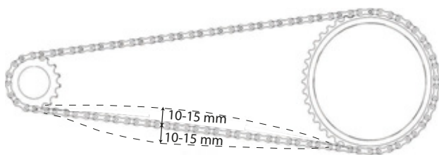
Figur 188: Kontrol af kædestramning
