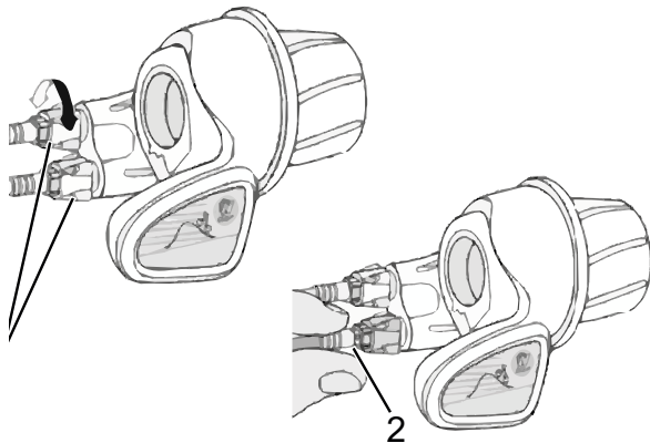
Figur 192: Drejegræb med slutmuffer (1) og slør i gearskifte (2)
