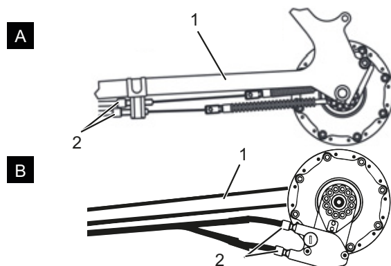
Figur 191: Slutmuffer (2) på to alternative udførelser (A og B) af et gearskifte med to kabler på baggafflen (1)
