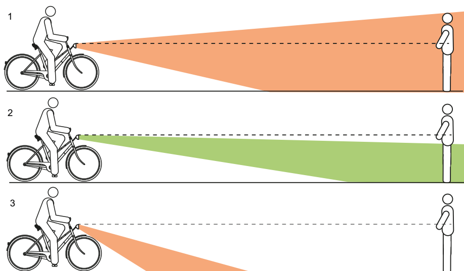
Figur 127: For højt (1), korrekt (2) og for lavt (3) indstillet lys
